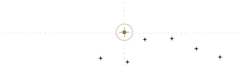
Triangulum Australe
