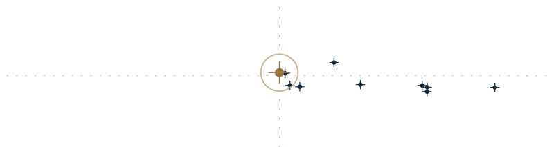
Piscis Austrinus
