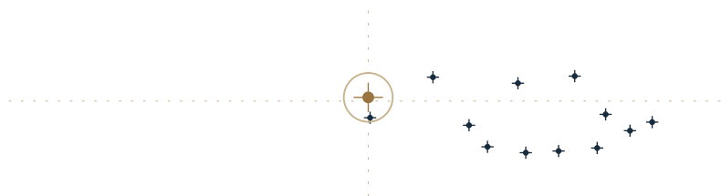
Corona Borealis
